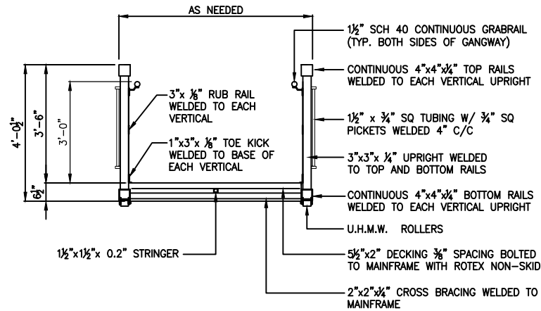
GANGWAY - SECTION
